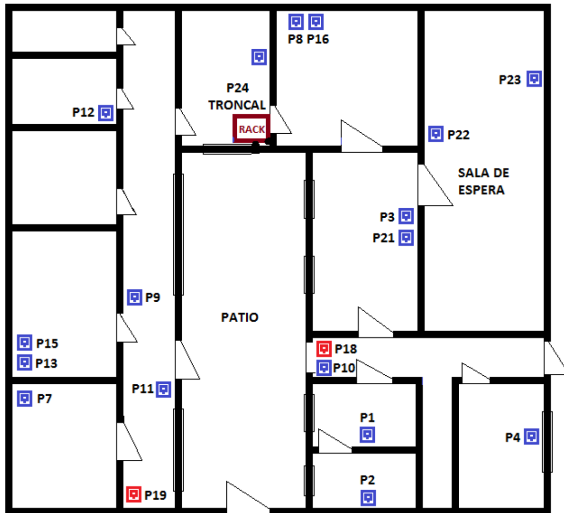
PLANTA BAJA
